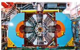
北京正负电子对撞机-谱仪全景
